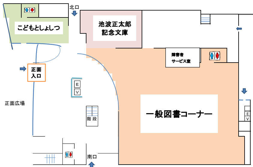
1階 平面図
